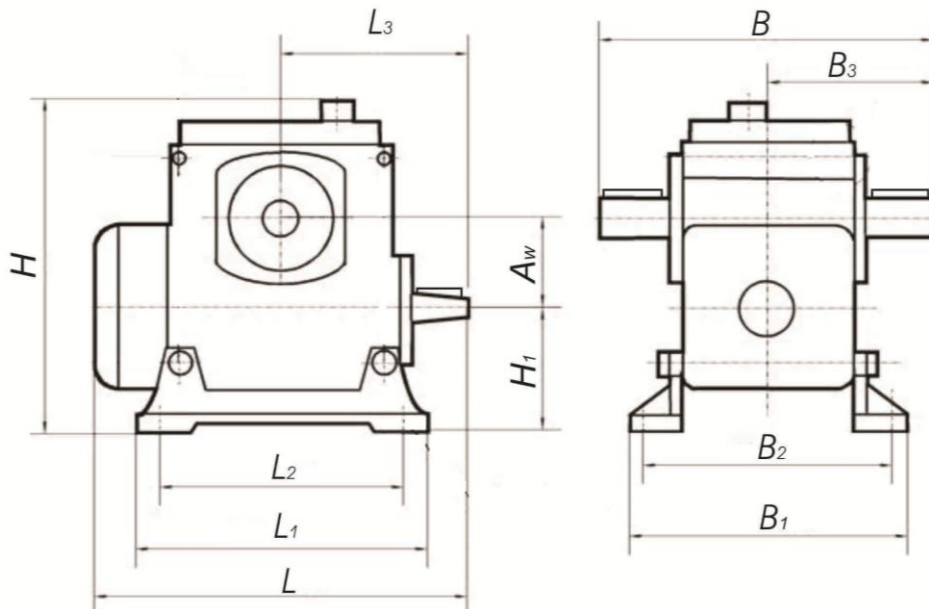
ГАБАРИТНЫЕ РАЗМЕРЫ РЕДУКТОРОВ Ч-80
